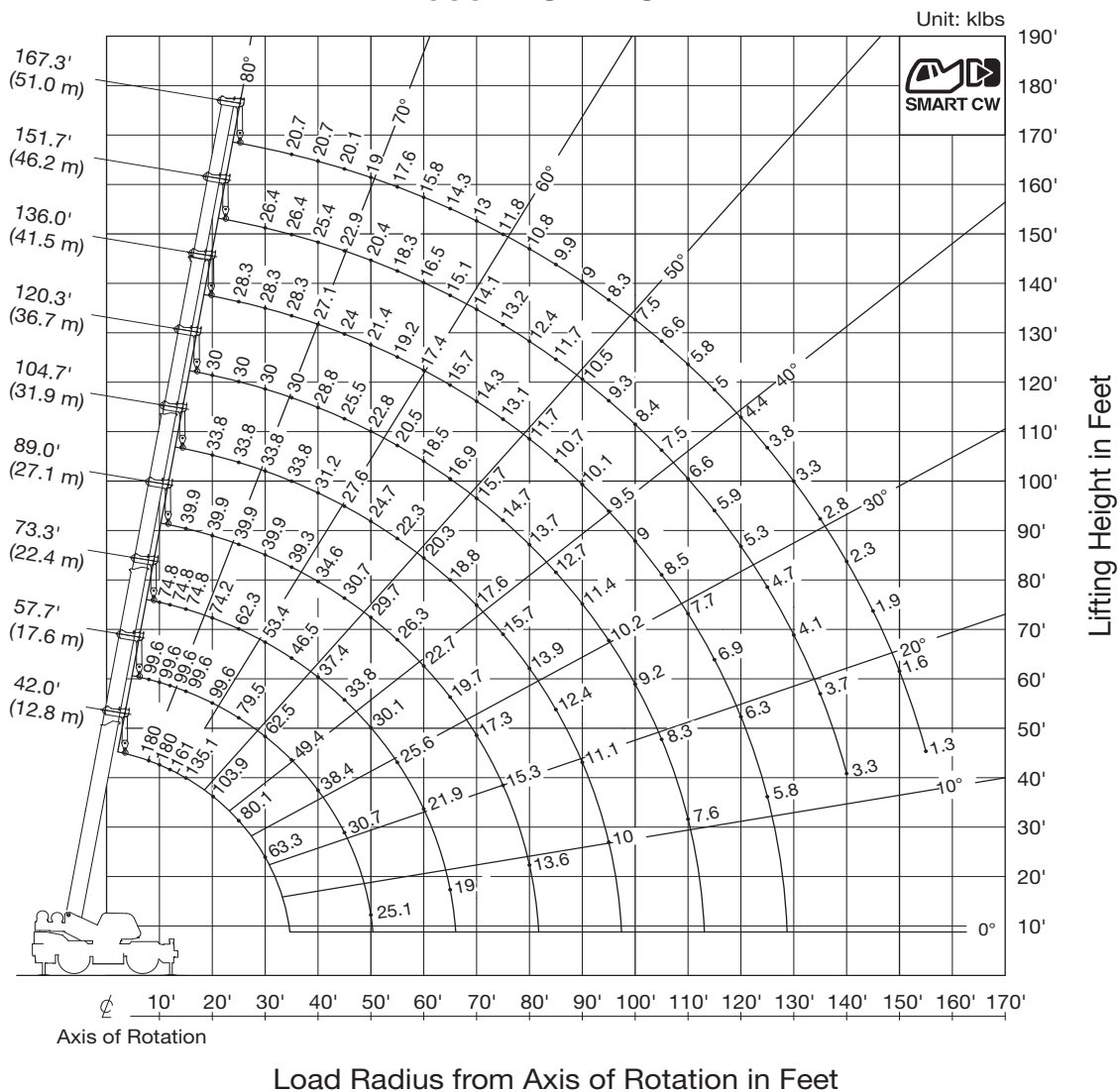
BOOM
